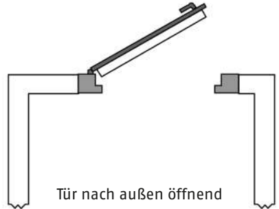
Stumpftür
